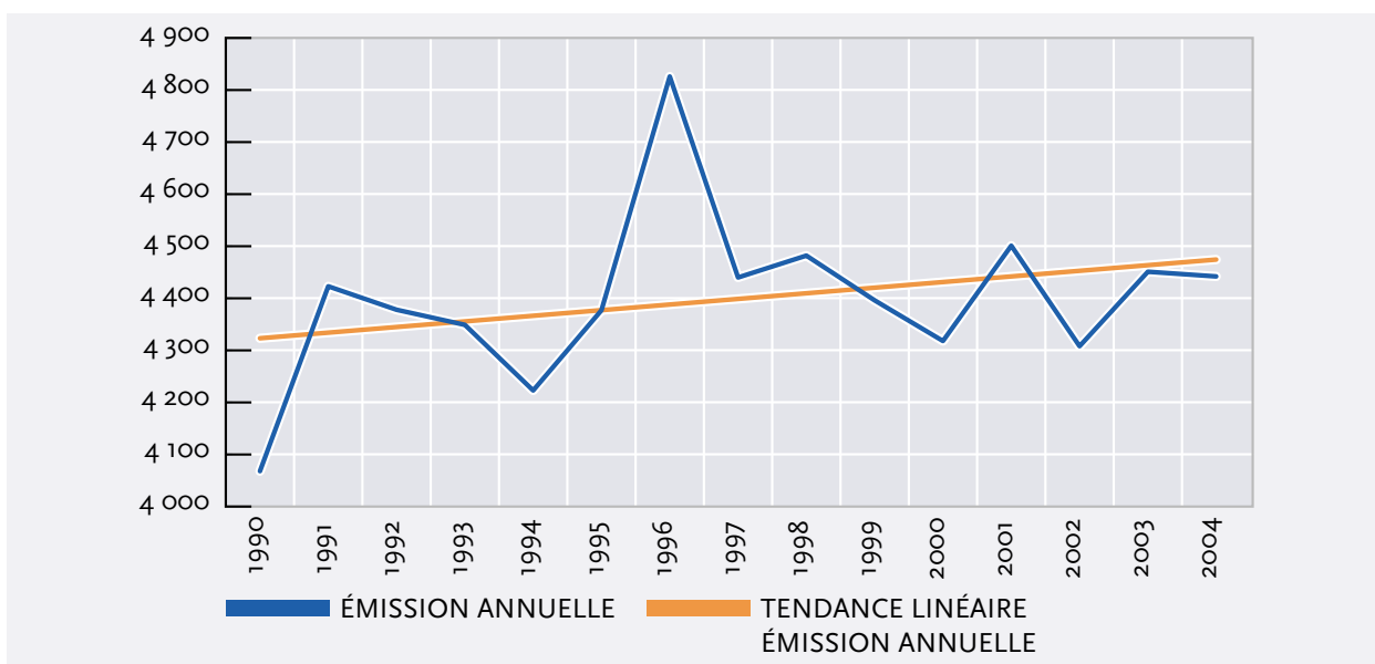
GRAPHIQUE 11: Émission de gaz à effet de serre en Région de Bruxelles-Capitale (en Kt d'équivalents CO 2 )
